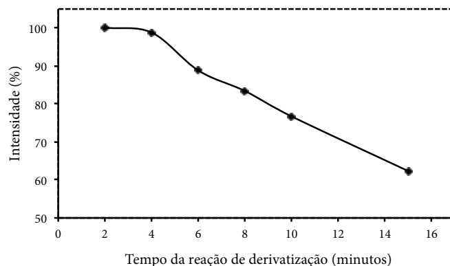
Figura 2. Fluorescência emitida pelo derivado fumonisina B 1 -orto-ftaldialdeído em diferentes tempos da reação de derivatização
