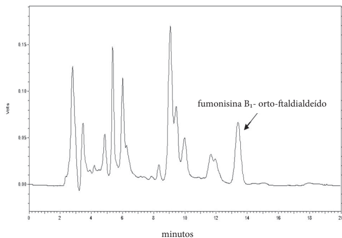
Figura 3. Cromatograma característico da separação e detecção do derivado fumonisina B 1 -orto-ftaldialdeído. Condições cromatográficas: fase móvel: acetonitrila; tampão fosfato de sódio 0,1 M pH 3,3 (44:56), vazão: 1,0 mL.min -1 , temperatura da coluna: 20 °C, volume injetado: 10 µL, e coluna ODS Hypersil de 250 × 4,6 mm d.i. e partículas de 5 µm
